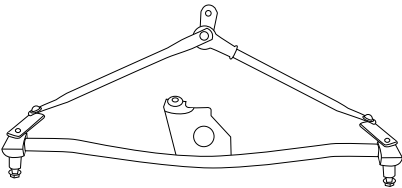
Трапеция стеклооч. для а/м KIA Rio II (VWA 0510)
