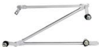
Трапеция стеклооч. для а/м Камаз Евро-2 (VWA 0702)
