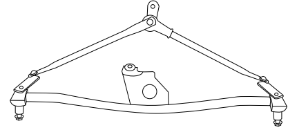
Трапеция стеклооч. для а/м Fiat/Sollers Ducato (02-14), Peugeot Boxer (02-14), Citroen Jumper (02-14) (VWA 1651)
